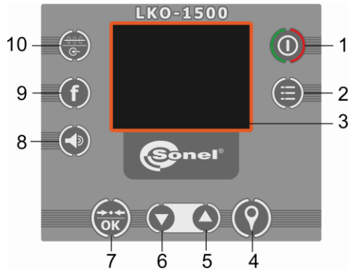
Fig. 9 Aspecto y marcaje de los botones del receptor LKO-1500
