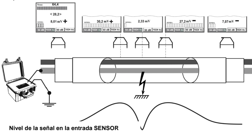
Fig. 33 Esquema de conexión del transmisor y la detección del lugar entre el conductor y el blindaje del cable
