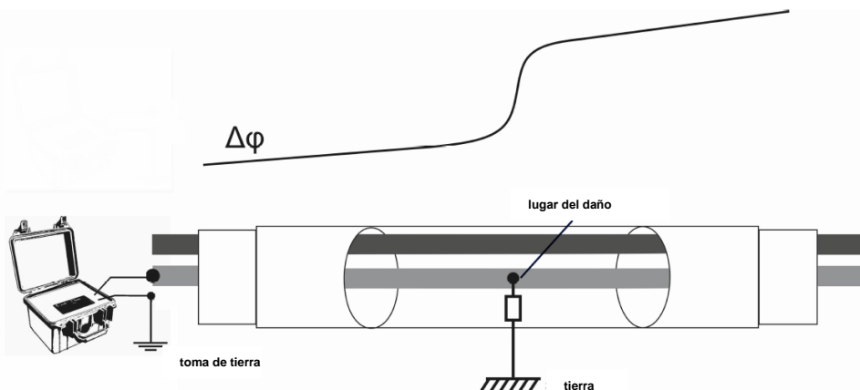
Fig. 34 Esquema de conexión del transmisor y el desplazamiento de fase durante la localización del daño de aislamiento usando el método de fase
