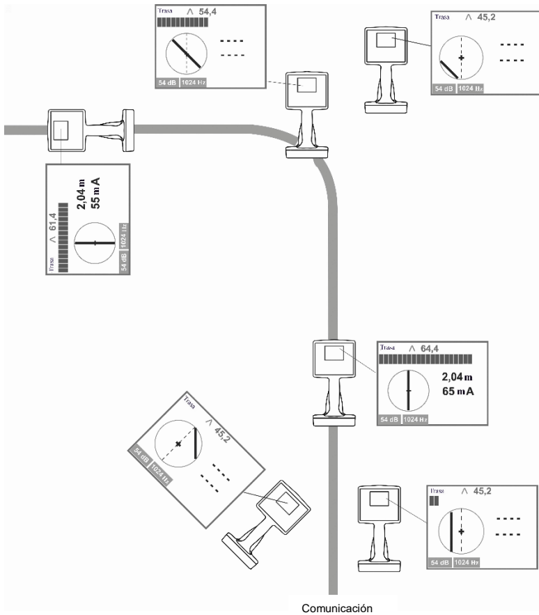
Fig. 23 Búsqueda con la opción "Brújula, línea"
