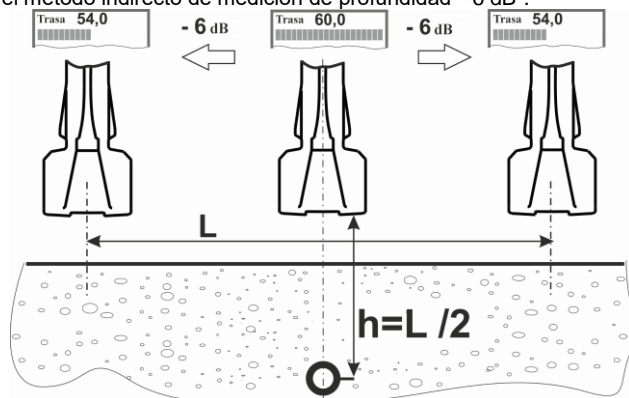
Fig. 27 Medición de profundidad con el método indirecto "-6 dB"
