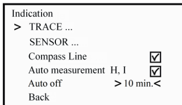
Fig. 11 Menú "Display"
