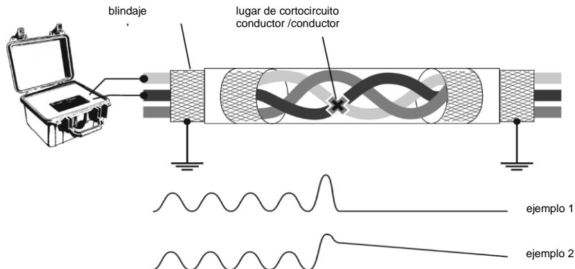
Fig. 31 Esquema de conexión del transmisor y la detección del lugar entre los conductores
