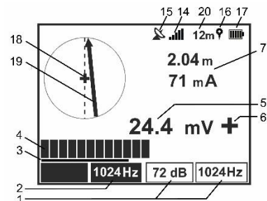
Fig. 21 Pantalla con brújula en modo "Trazado-SENSOR"
