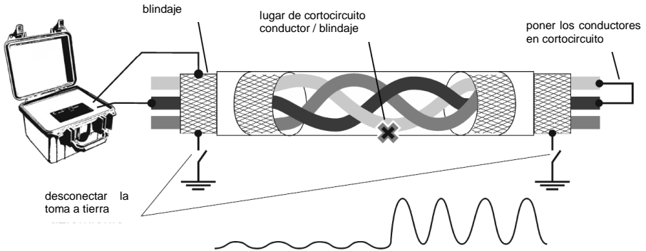
Fig. 32 Esquema de conexión del transmisor y la detección del lugar entre el conductor y el blindaje del cable
