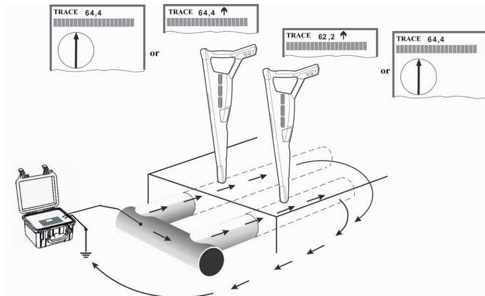
Fig. 25 Dirección de flujo de la corriente en los tubos conectados galvánicamente
