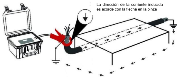
Fig. 6 Excitación inductiva de la corriente en el objeto examinado con la pinza N-1
