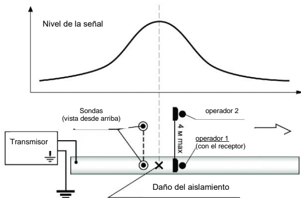
Fig. 30 Detección de daños en el aislamiento con el método de aumento de la señal
