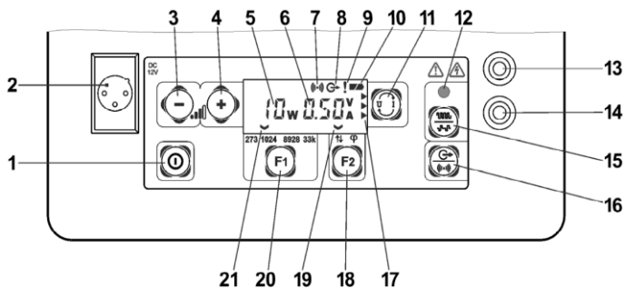
Fig. 2 Panel frontal del transmisor LKN-1500
