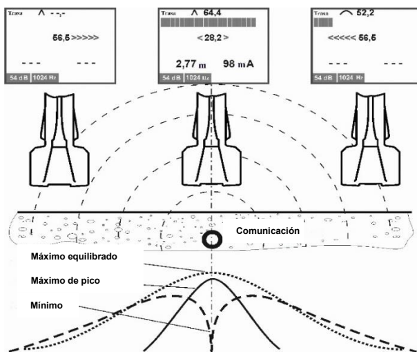
Fig. 22 Cambio de nivel de la señal con el desplazamiento del receptor hacia un lado del trazado de la línea
