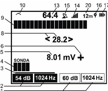
Fig. 20 Pantalla en modo "Trazado-SENSOR"
