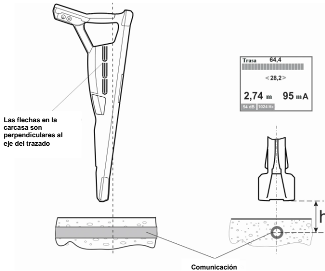
Fig. 26 Medición directa de la profundidad
