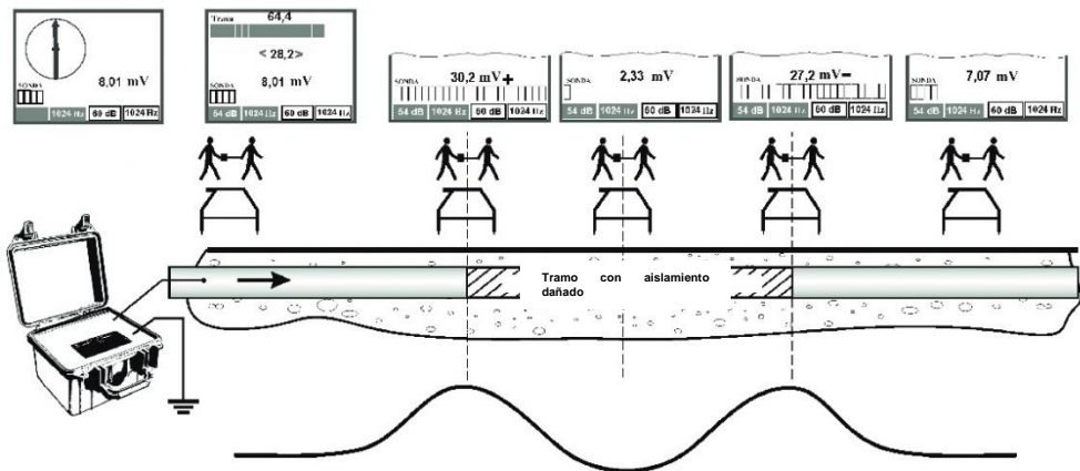
Fig. 29 Localización de daño con el metodo de caída de tensión.
