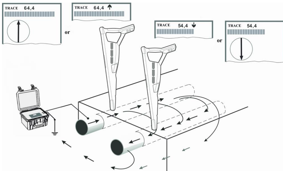
Fig. 24 Dirección del flujo de corriente a través de la línea adyacente, sin conexión galvánica
