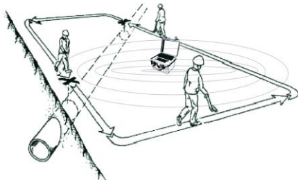
Fig. 28 Estudio del área utilizando el transmisor en modo inductivo
