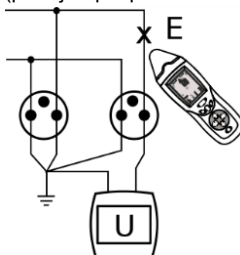
Fig. 8 Esquema del modo de tensión.
