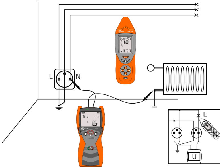
Fig. 24 Localización de conductores en la pared desconectados de la red.
