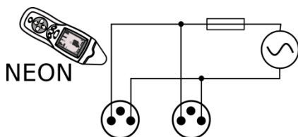
Fig. 14 Esquema del modo de detección del campo eléctrico de 50Hz/60Hz.
