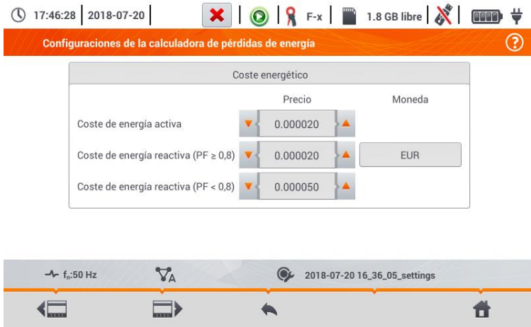
Fig. 5.30 Análisis de las pérdidas de energía - pantalla de configuración 2
