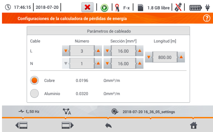
Fig. 5.29 Análisis de las pérdidas de energía - pantalla de configuración 1
