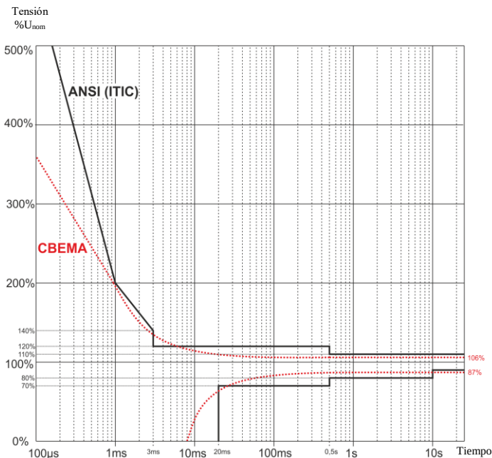
Fig. 21. Curvas de tolerancia de tensión de alimentación ANSI (ITIC) y CBEMA.
