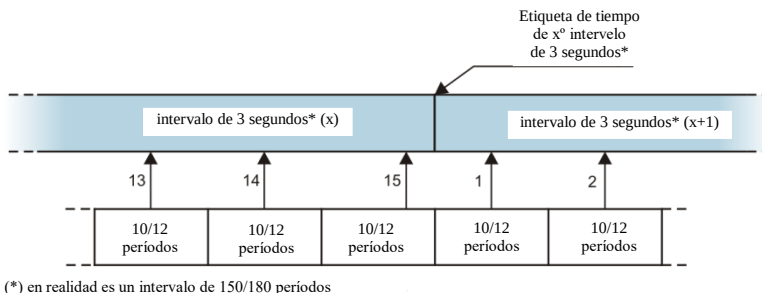
Fig. 23. Determinación de intervalos de cálculo de media más cortos que 10 segundos (por ejemplo para el cálculo de promediación de 3 segundos)
