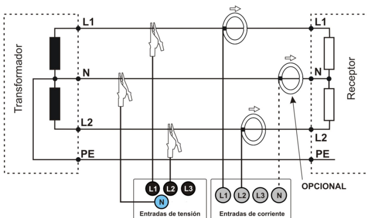
Fig. 6. Esquema de conexión – sistema bifásico.
