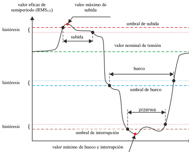
Fig. 19. Subidas, huecos e interrupciones de tensión.
