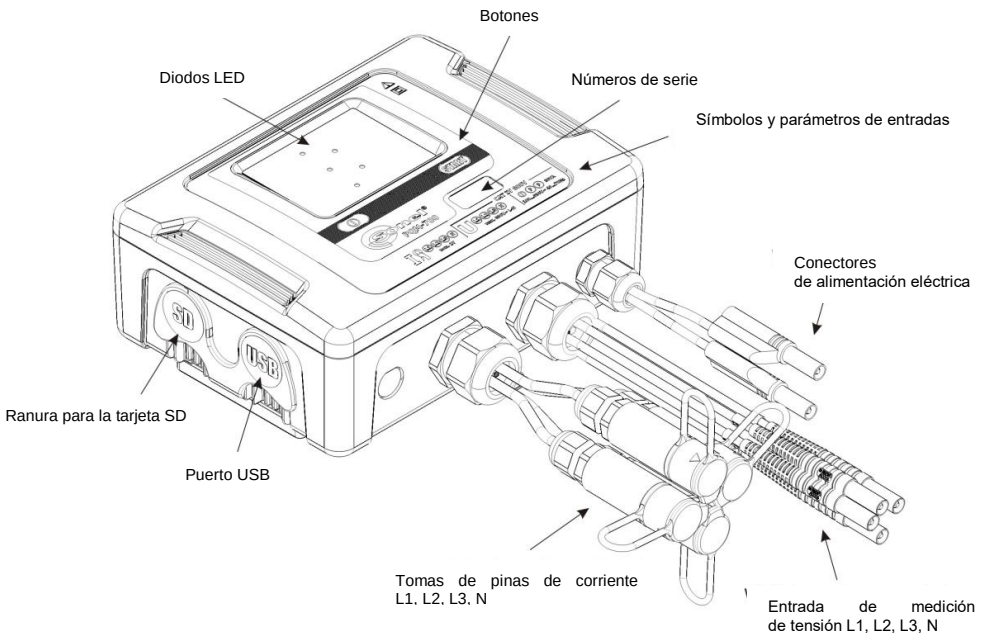
Fig. 1. Analizador de calidad de energía eléctrica PQM-700. Vista general.
