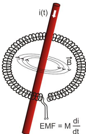
Fig. 17. Bobina de Rogowski
