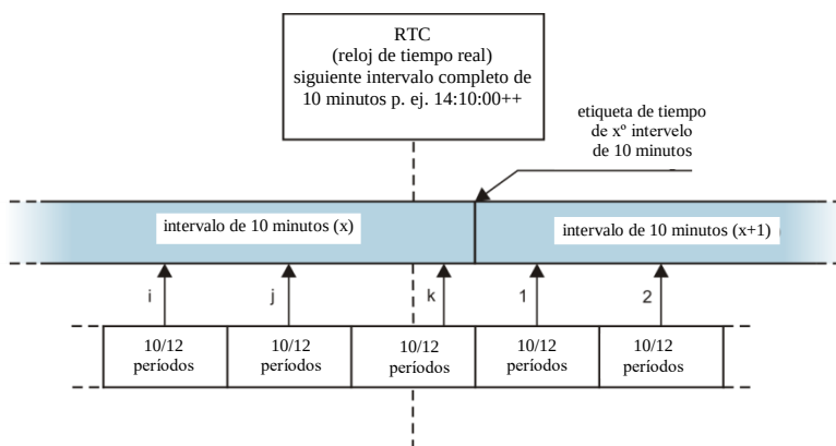
Fig. 22. Determinación de períodos del cálculo de media más largos (o iguales) a 10 segundos (por ejemplo para 10 minutos)
