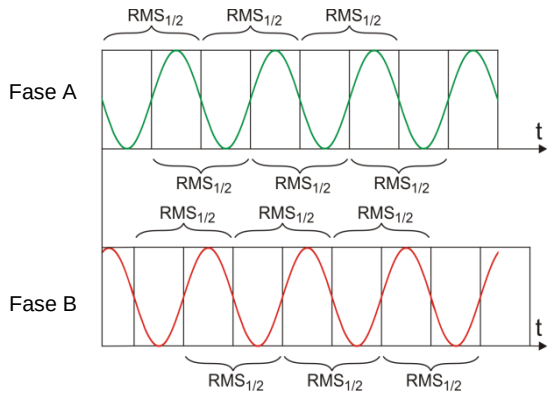
Fig. 20. Determinación del valor U_{RMS(1/2)}
