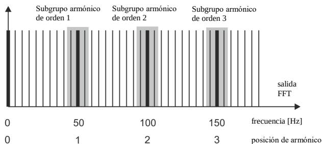
Fig. 15. Determinación de subgrupos de armónicos (red de 50 Hz).
