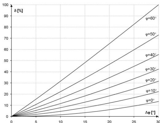
Fig. 24. La incertidumbre adicional resultante del error de fase, dependiendo del ángulo de desplazamiento de fase.
