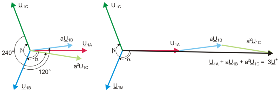
Fig. 18. Ejemplo de determinación de componente de secuencia positiva.
