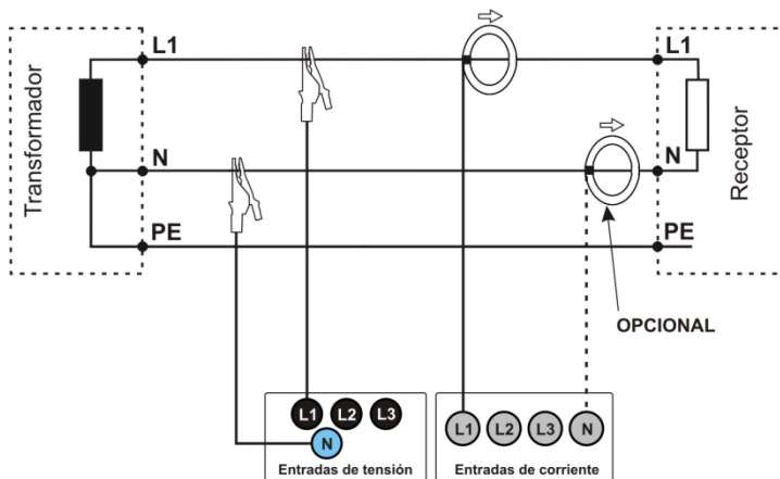
Fig. 5. Esquema de conexión – sistema monofásico.
