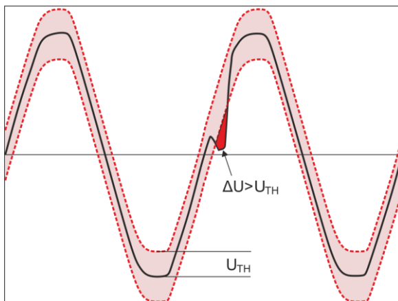
Fig. 42. Detección de eventos por el cambio de forma de la envoltente.
