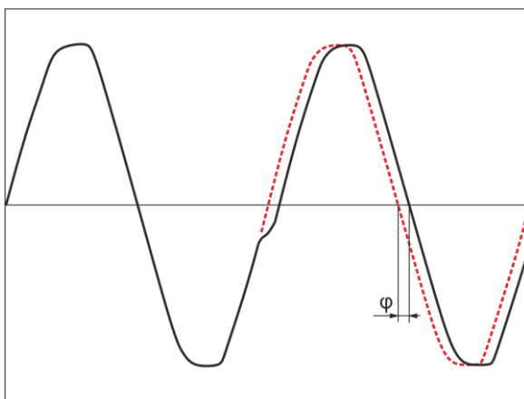
Fig. 43. Salto de la fase.
