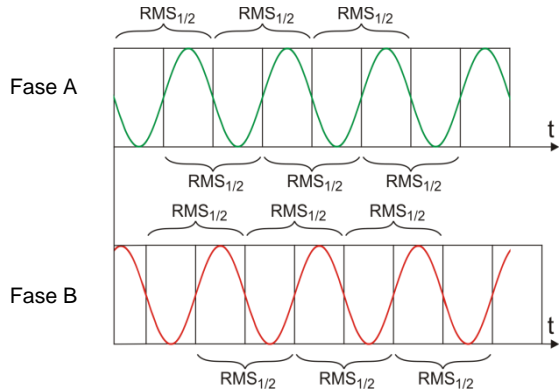
Fig. 52. Determinación del valor U_{RMS(1/2)}
